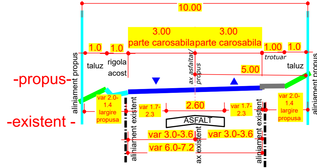
PROFIL TRANSVERSAL CARACTERISTIC c-c scara 1:100
