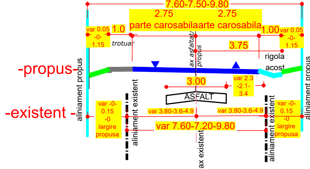
PROFIL TRANSVERSAL CARACTERISTIC b-b scara 1:100
