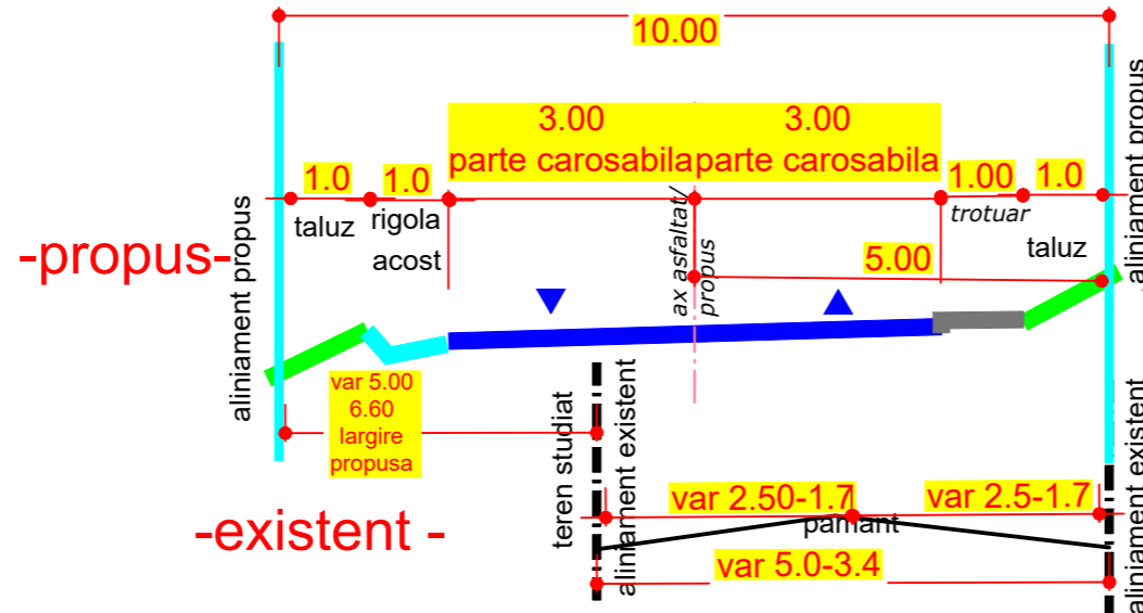
PROFIL TRANSVERSAL CARACTERISTIC d-d scara 1:100
